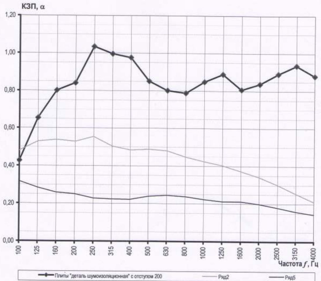
Рисунок 1 – Реверберационный коэффициент звукового поглощения испытанного образца № 1
